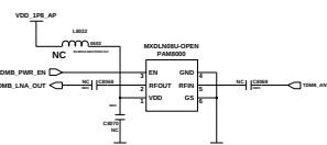
TDMB LNA
